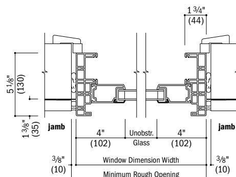
Horizontal Section Patio Door Sidelight/Transom
