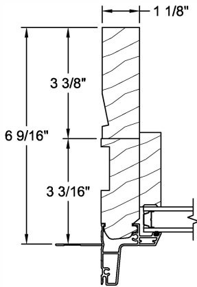
6 9/16" Jamb Width 5/4 Jamb Thickness
