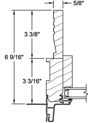
6 9/16" Jamb Width 4/4 Jamb Thickness
