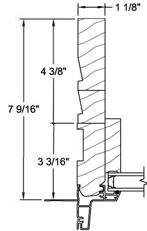
7 9/16" Jamb Width 5/4 - 5/4 Stacked Jamb
