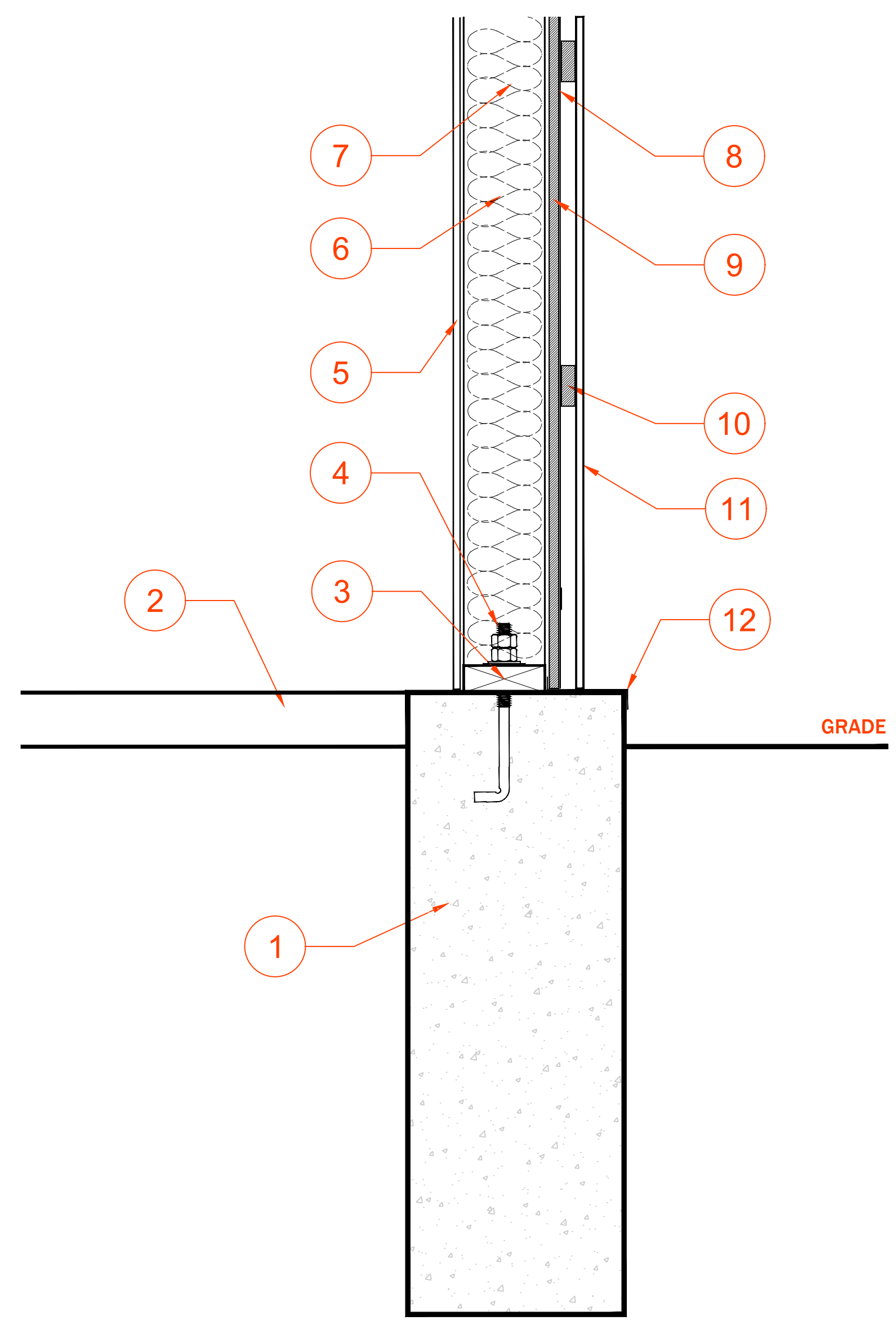
ws Wall section Scale: 1/8"=1'-0"
