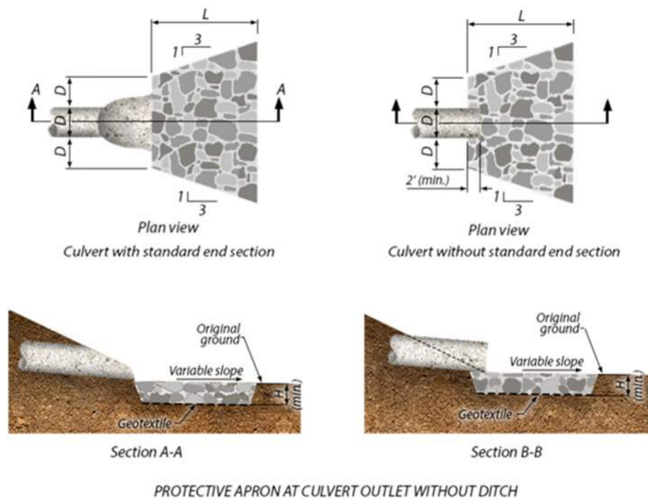
Figure 5-12 Riprap Apron
