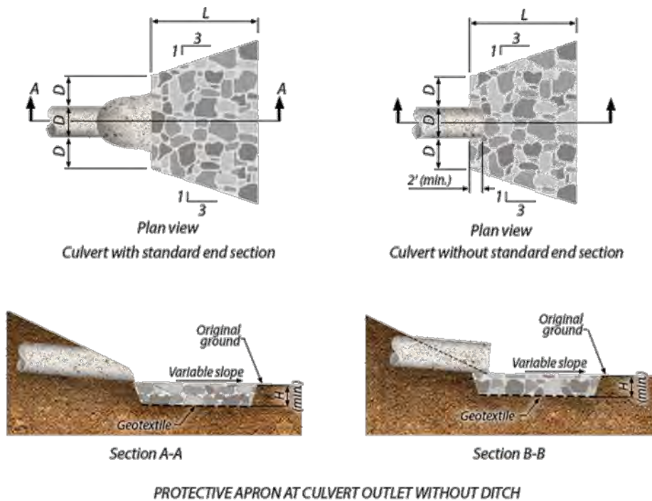
Figure 5-12 Riprap Apron
